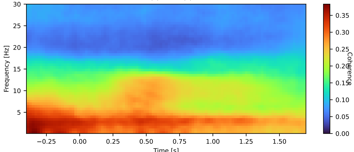
8B (1) - dPFC (4)
